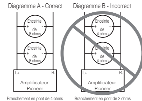
Branchement en pont de 4 ohms Branchement en pont de 2 ohms
