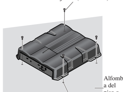
Perfore un orificio de 2,5 mm de diámetro
