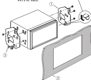
Vis à tête bombée (5 mm x 8 mm) (6 pièces)
